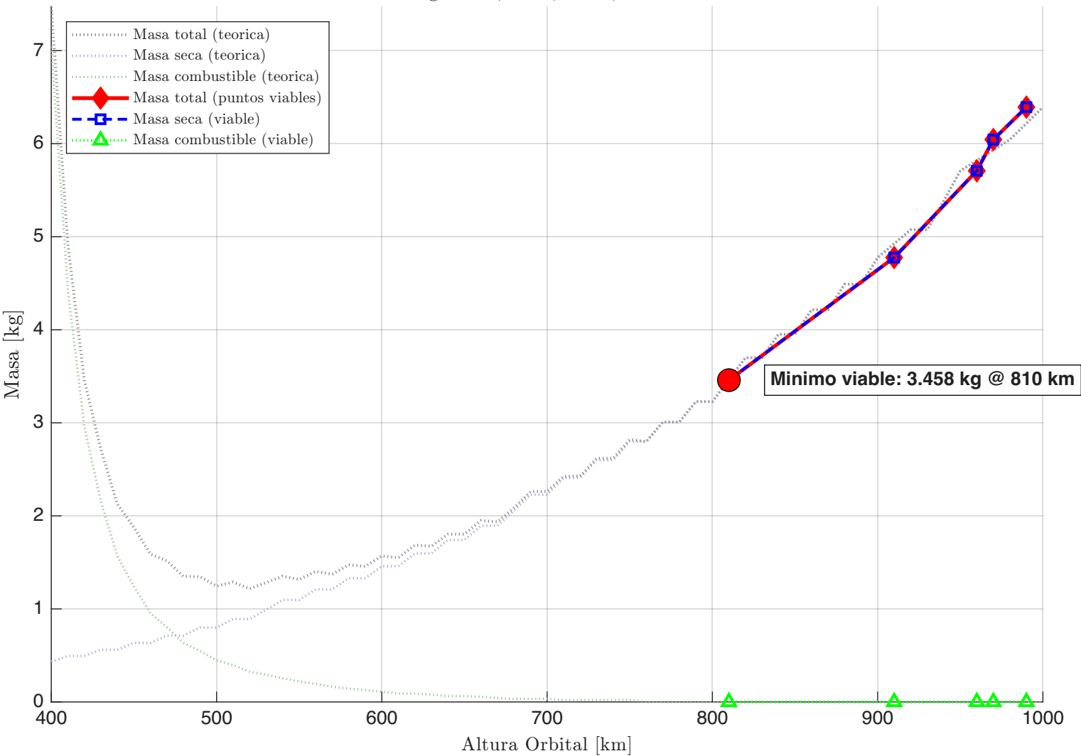
Desglose de Masas vs. Altura Config: 3 Sat, 1 Tel, Det 2, Refractivo
